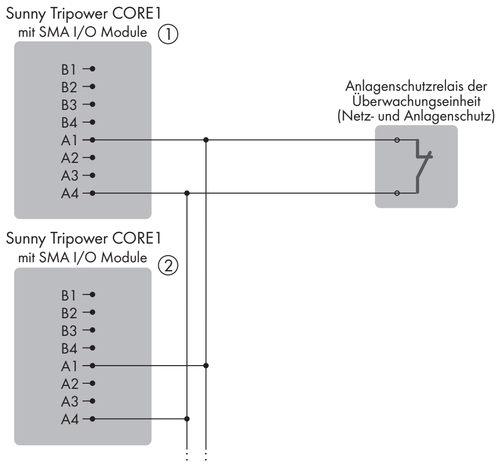
Abbildung 4: Verdrahtungsbeispiel für Netz- und Anlagenschutz ohne Wirkleistungsvorgabe
