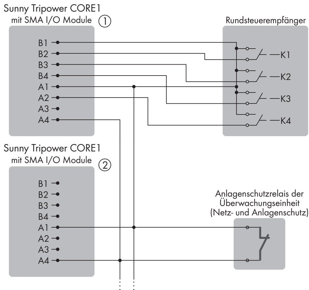
Abbildung 5: Verdrahtungsbeispiel für Netz- und Anlagenschutz mit Wirkleistungsvorgabe
